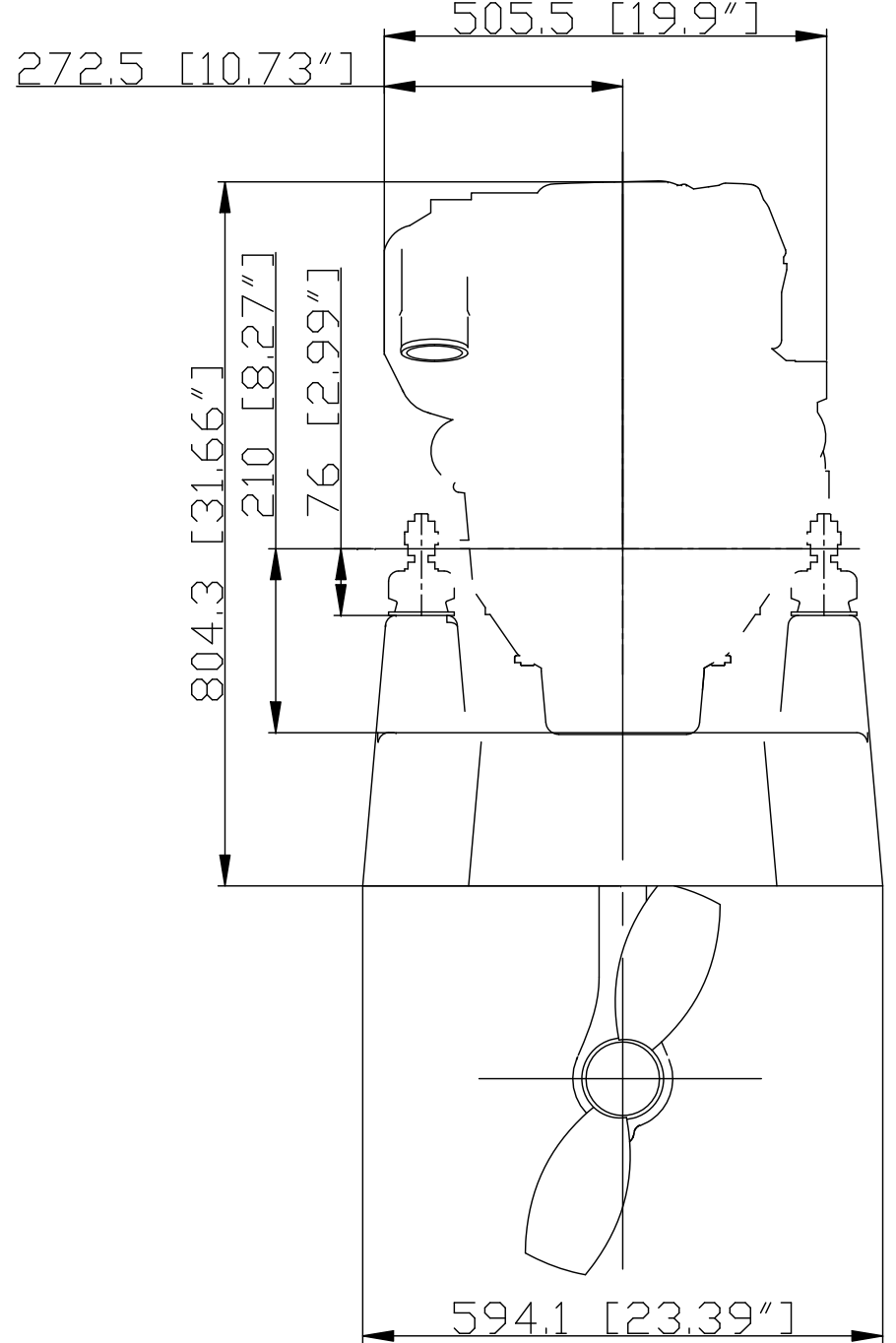
N4.60 SAIL DRIVE PLAN D'ENCOMBEMENT Ech. 1/10 Le 11-05-05
