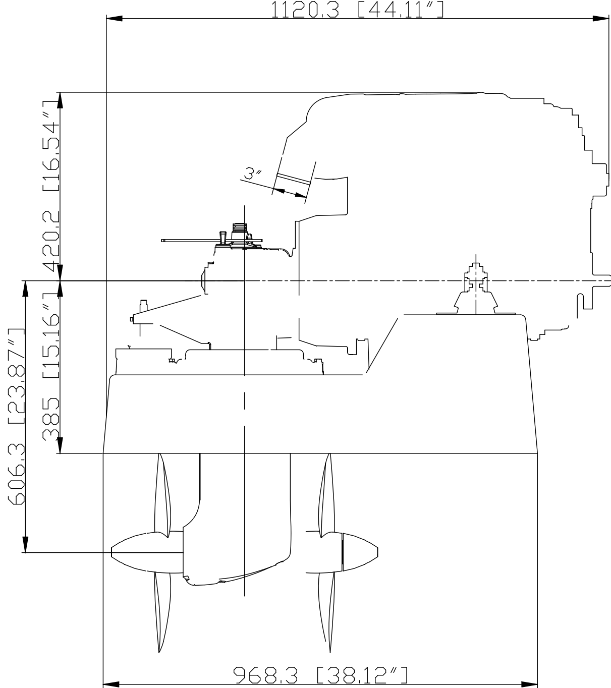
N4.60 SAIL DRIVE PLAN D'ENCOMBEMENT Ech. 1/10 Le 11-05-05
