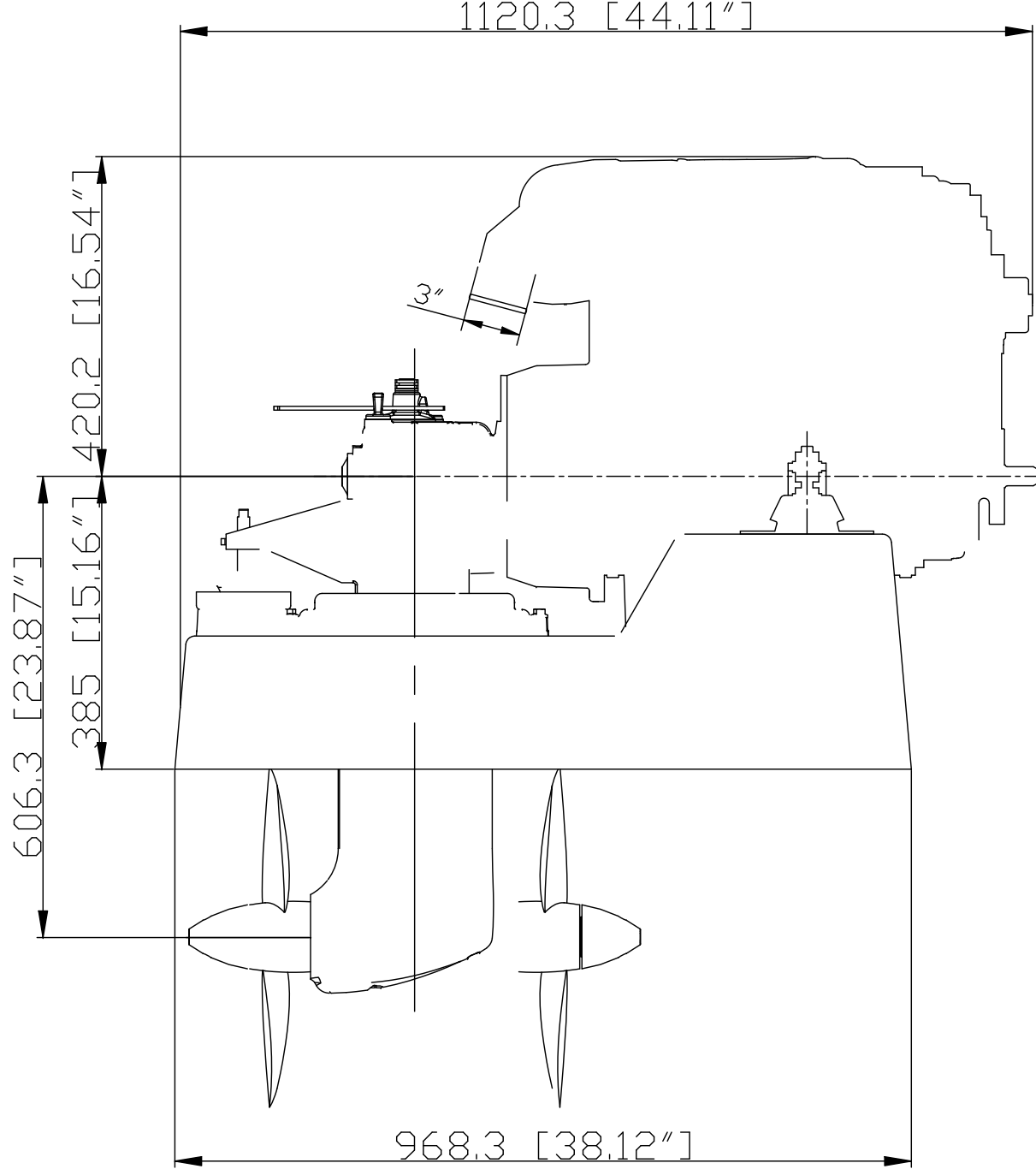
N4.60 SAIL DRIVE PLAN D'ENCOMBREMENT Ech. 1/10 Le 11-05-05
