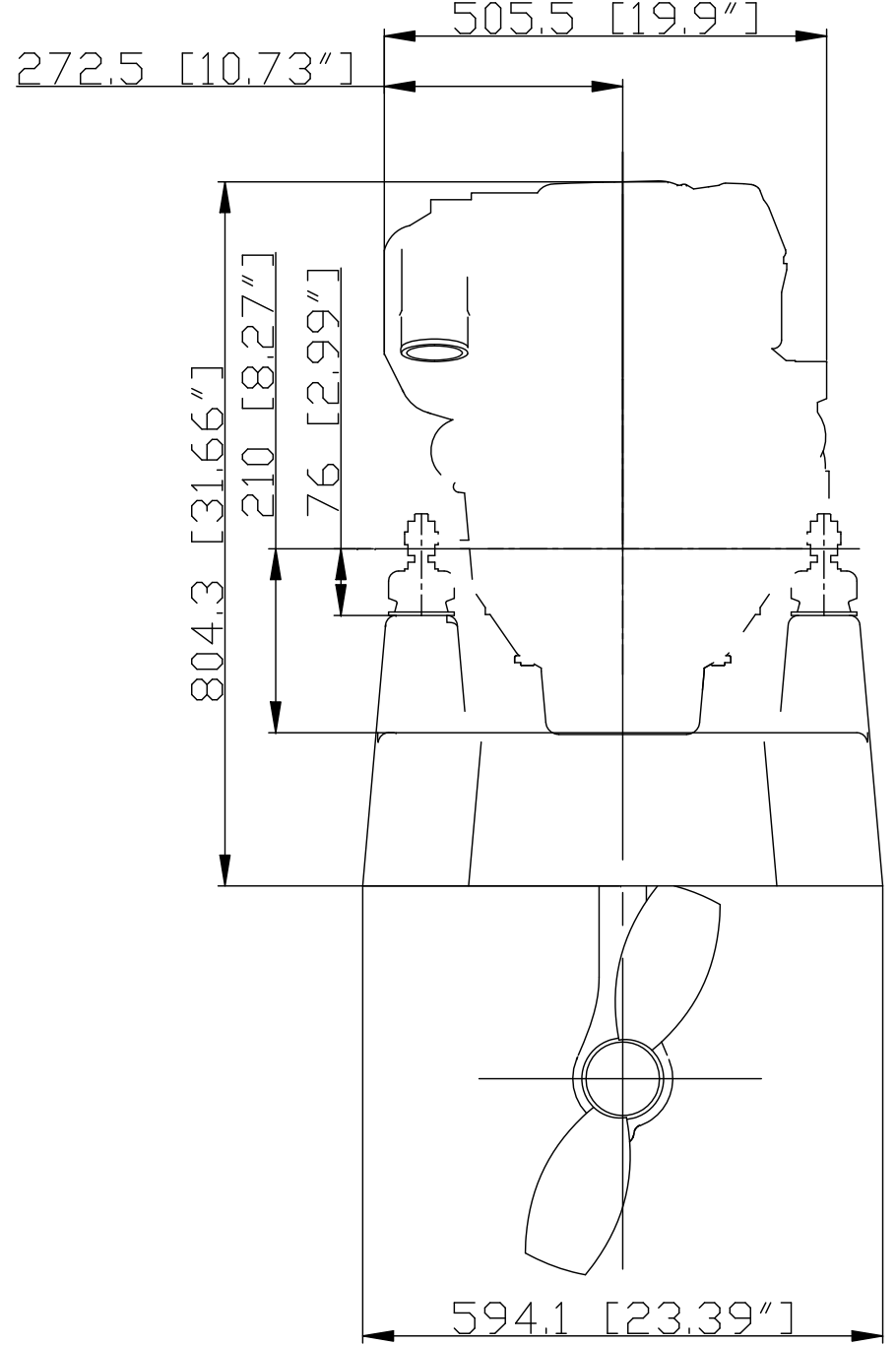
N4.60 SAIL DRIVE PLAN D'ENCOMBREMENT Ech. 1/10 Le 11-05-05
